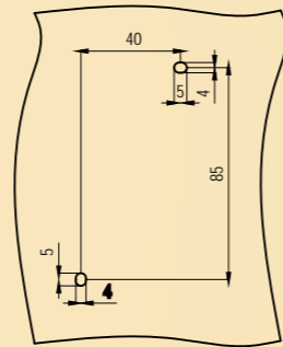
螺钉安装尺寸
