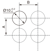
□ K10安装尺寸 / K10 Installation size
