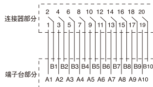
接线图
