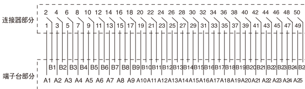
接线图
