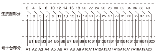
接线图
